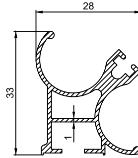
P.No 2858 0.406 Kg/m
