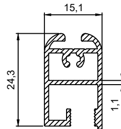
P.No 3202 0.316 Kg/m
