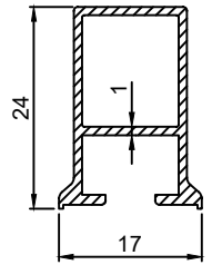
P.No 2859 0.228 Kg/m
