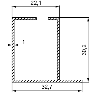
P.No 2887 0.286 Kg/m
