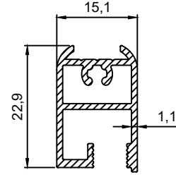
P.No 3638 0.285 Kg/m
